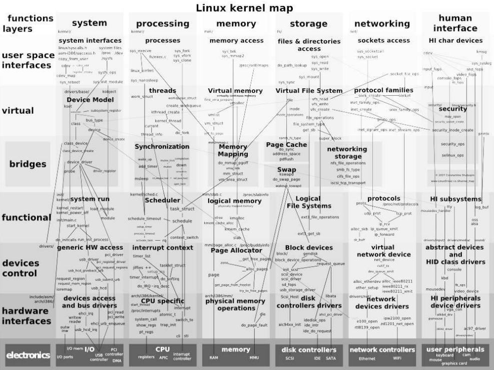
Linux kernel map.
